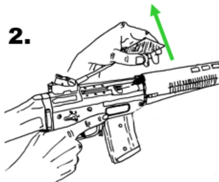
2. Levare il parabossoli
