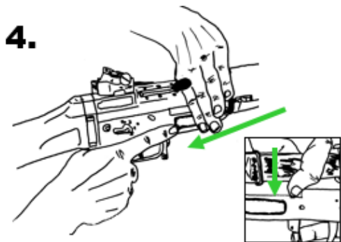
4. Arretrare l'otturatore e bloccarlo
