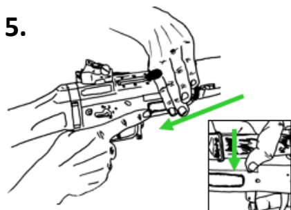
5. Arretrare l'otturatore e bloccarlo
