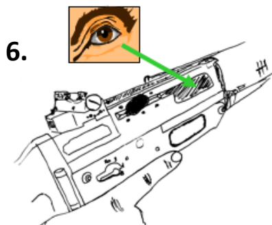
6. Controllare la camera delle cartucce
